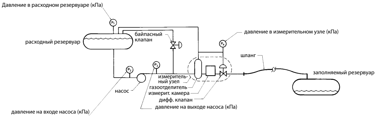
Принципиальная схема насосной системы
