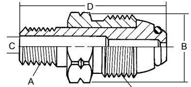
970S (CGA 510) POL Соединение POL с отв. 60 DMS и мягким носком
