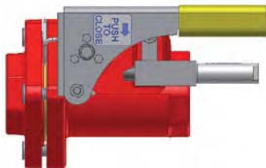
Модель 6016 с устройством пневмоконтроля 6016-60D
