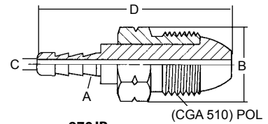
970JR (CGA 510) POL Соединение POL с жестким носком
