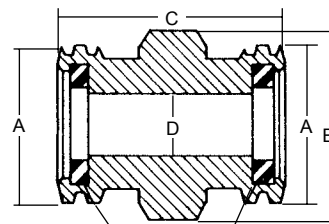
уплотнители в разъеме ACME x ACME
