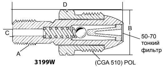
3199W (CGA 510) POL Усиленное соединение POL с жестким носком и скоростным клапаном
